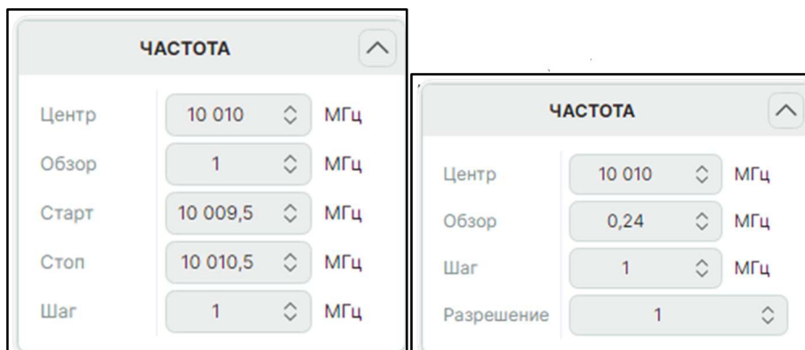
Рисунок 16 – Пример панели управления «Частота»:
